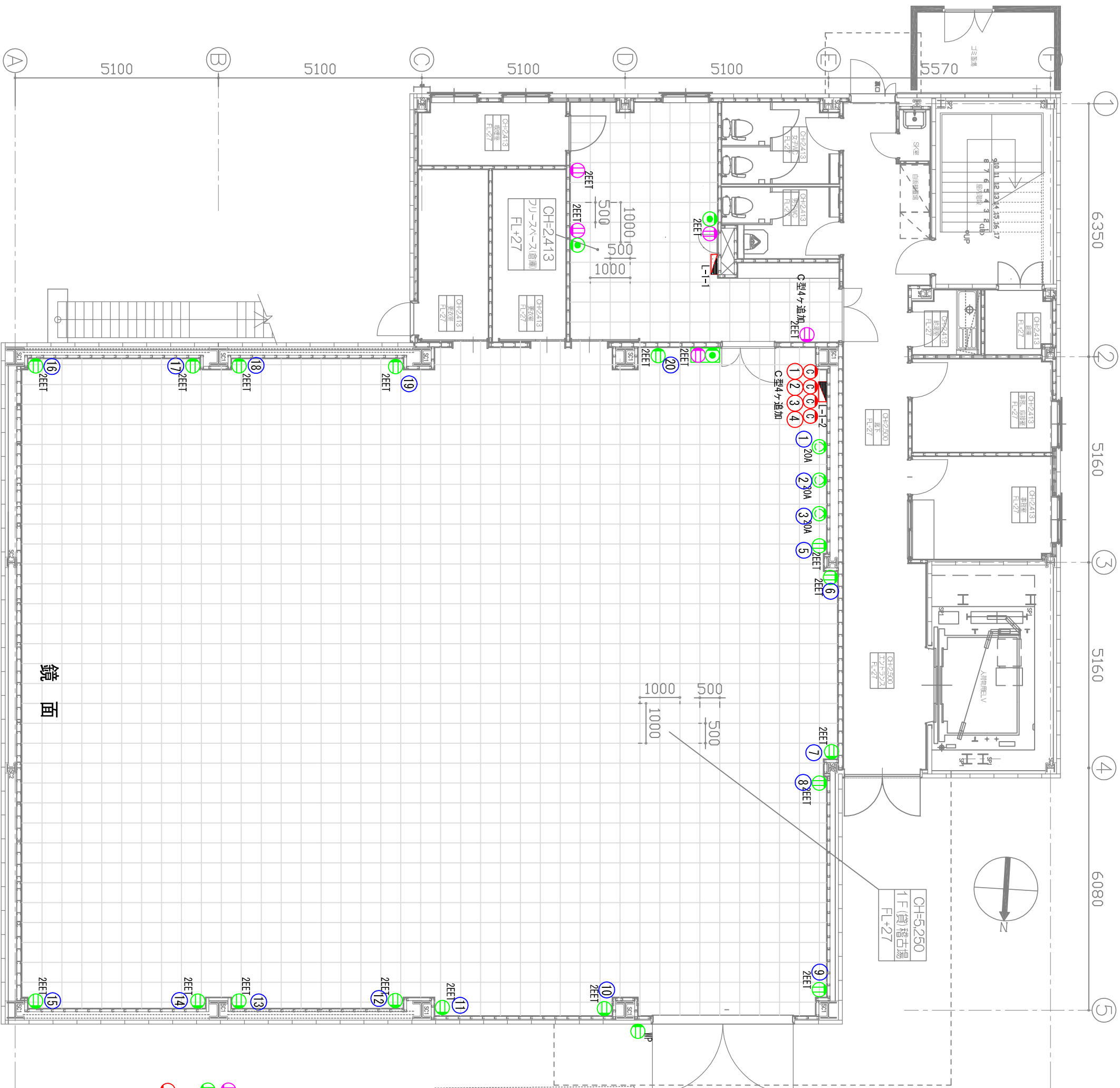
明治座森下スタジオ 1F平面図 1/100
